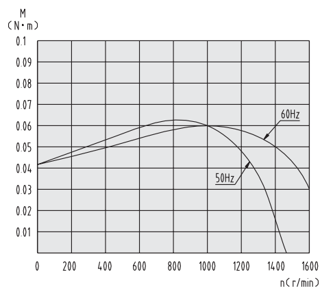
转矩-转速曲线
